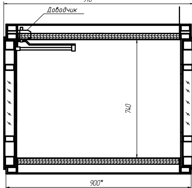
Б-Б
